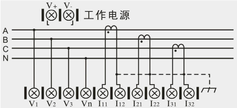
图 5.3 三相四线(无 PT)接线图
